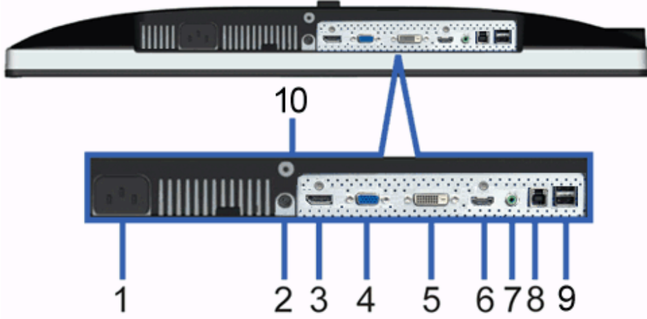
Altan görünüm
